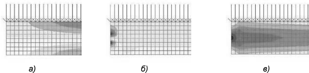
Рис. 4 Поля напружень в приопорній зоні балки Б-1: а) \sigma_x ; б) \sigma_y ; в) \tau_{xy}
